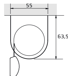
Kattokiinnitys
